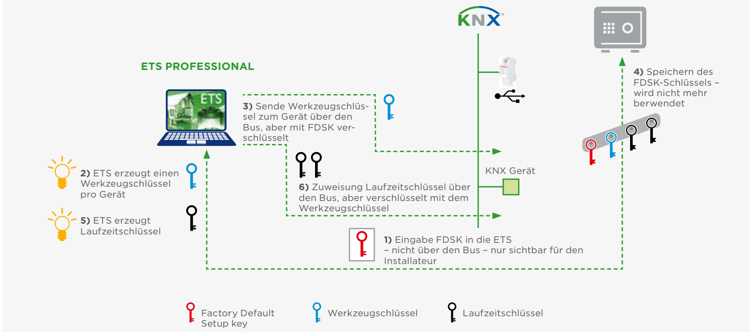
Verfahren zu Verschlüsselung von KNX Geräten
