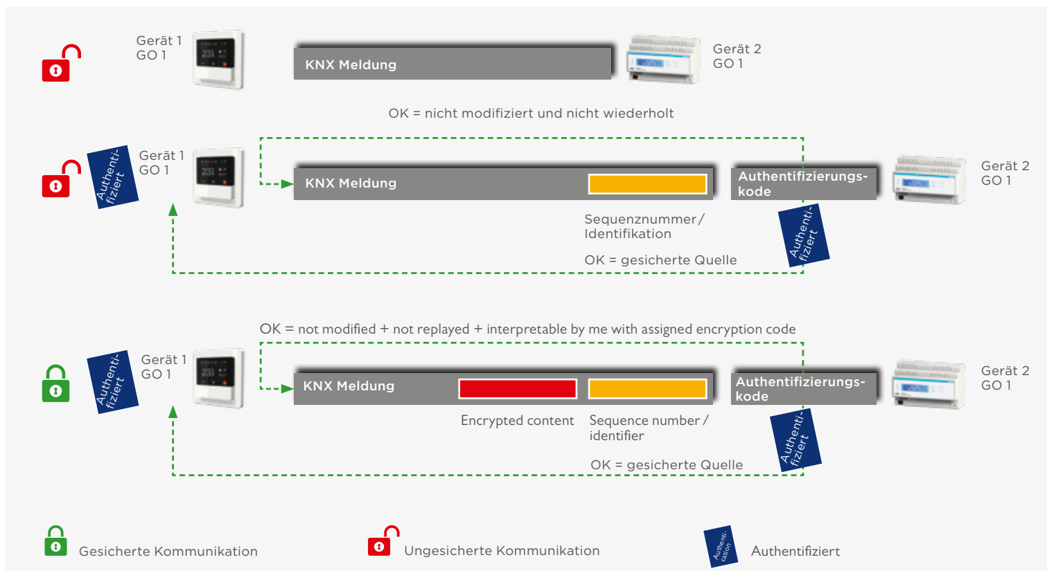
Übersicht der KNX Data Security Mechanismen
