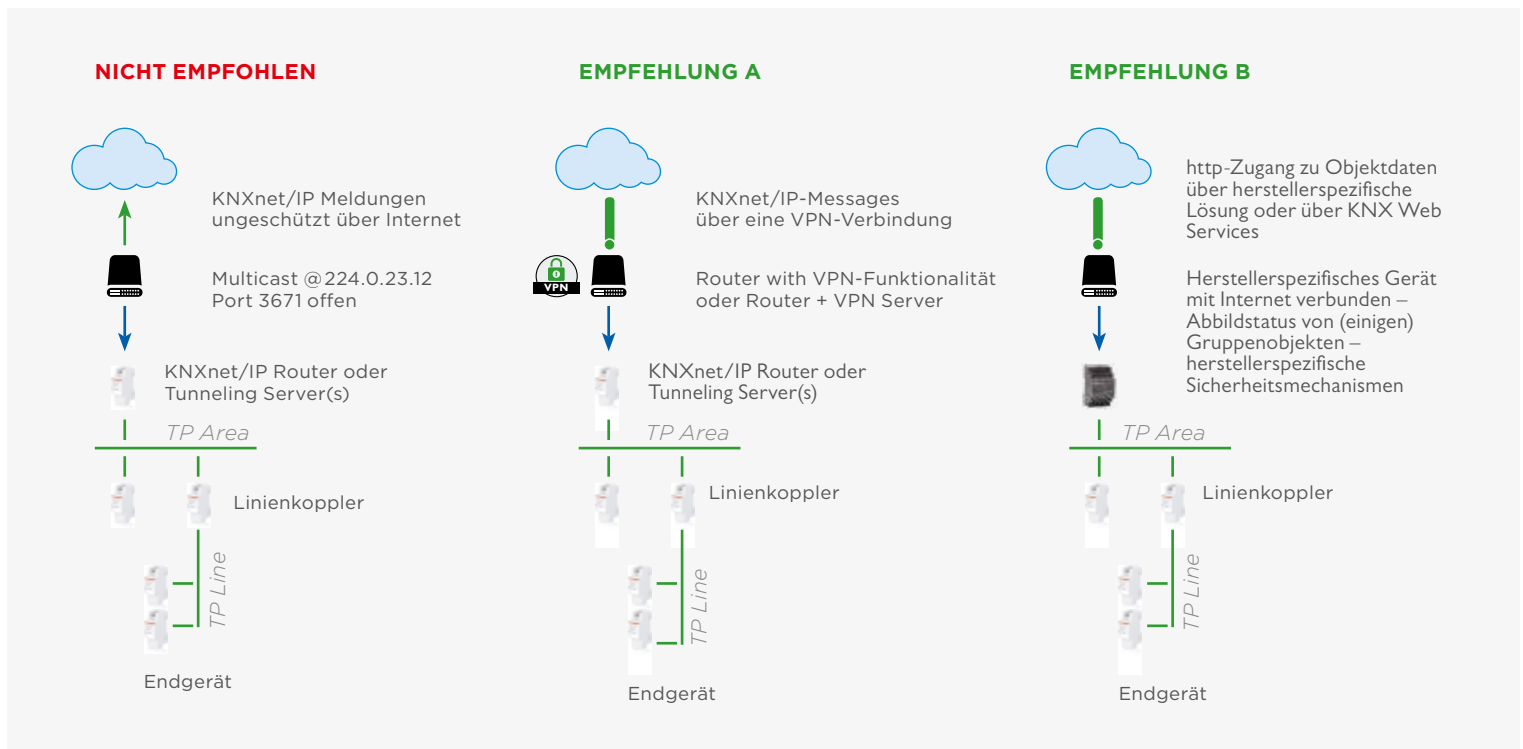
Zugang zu KNX Netzwerken über Internet
