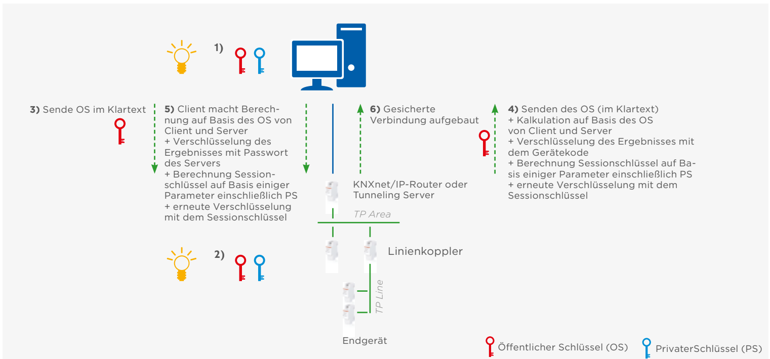
Aufbau einer KNX IP Secure Verbindung
